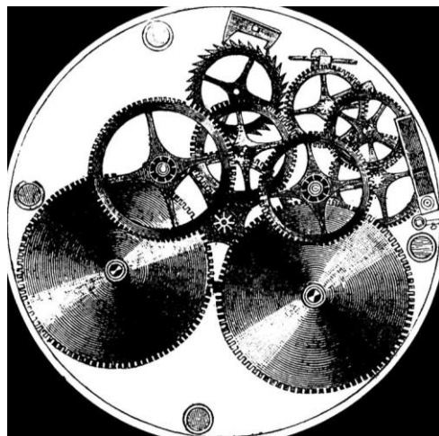
Ci-dessus : rouage de pendule d'appartement. Extrait des Arts et métiers illustrés d'A. Bitard (s.d.).
