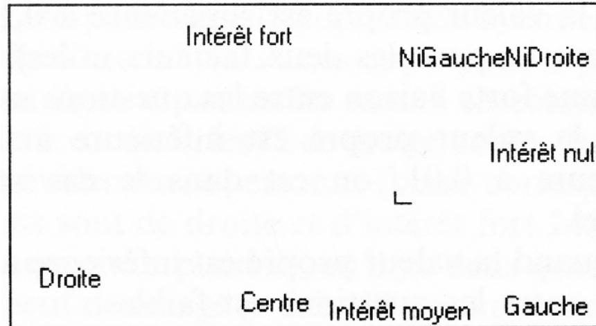
Fig. 2. – Plan factoriel du tableau de Burt, facteur 1 horizontal, facteur 2 vertical
