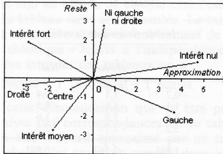
Fig. 1. – Facteur approximation en abscisse, reste en ordonnée
